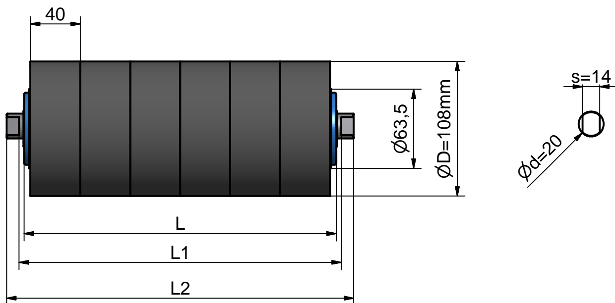
STANDARDNÍ ROZMĚRY
